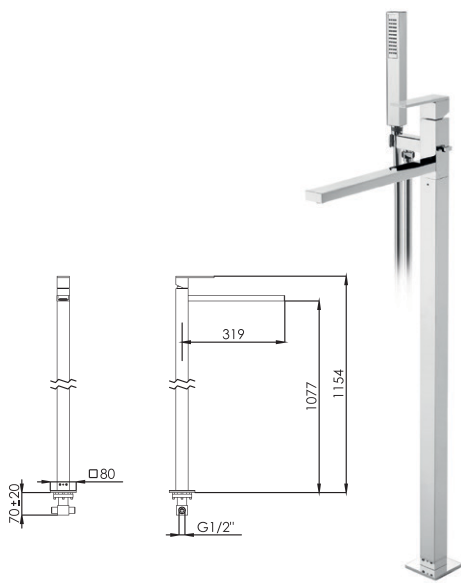
ASM-E550 MONOC. ESQUADRO BANHEIRA AO CHÃO
